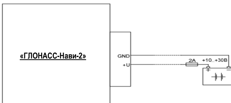
Рис. 2. Типовая схема подключения питания терминала.
