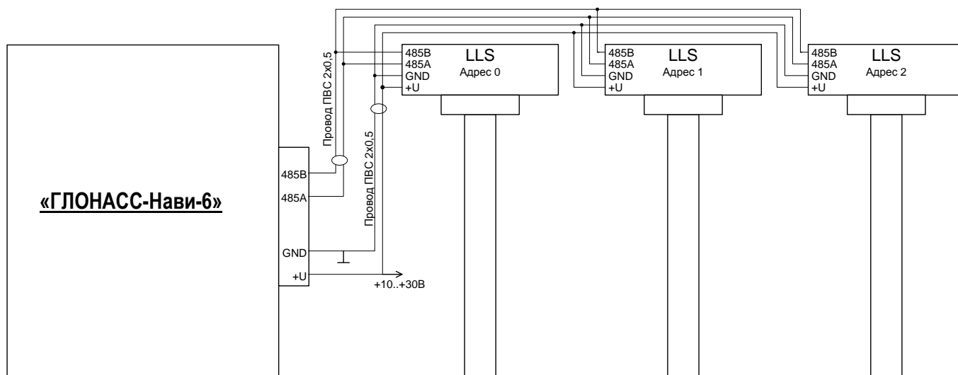
Рис. 3. Схема подключения датчиков уровня топлива LLS по интерфейсу RS485.
